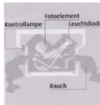
Vereinfachte grafische Darstellung der Rauchmesskammer eines Melders im Bereitschaftszustand und bei Raucheintritt.
